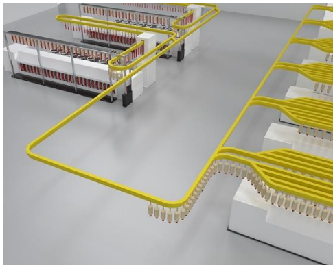
环锭纺中 Autoflow 系统
