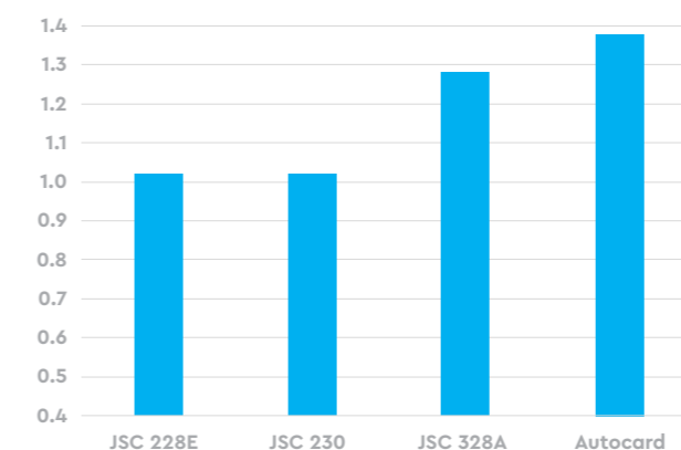
梳理宽度 以米为单位
